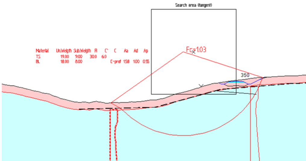
Figur 4-19: Utlipp fra beregning av stabilitet ned mot dalbunnen ved ca. profil 350 for alternativ C006. Alternativene C005 og C006 er forholdsvis like.
