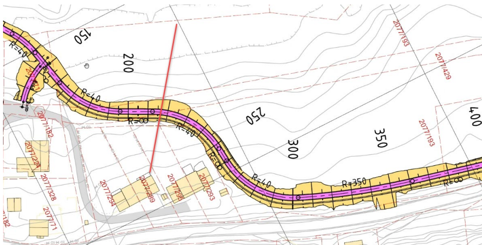
Figur 4-12: Plantegning med g/s-vei på vestsiden av Dalveien 36 og 38, her vist for alternativ C009, ved profil 230. Profilsnittet er angitt med rød linje.
