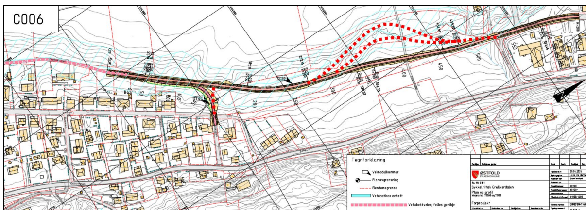
Figur 7-12: Forslag til optimalisering av alternativ 6. Rødstiplede linjer viser alternative traseer som bedre ivaretar dyrka mark og geoteknikk. (Kilde: ØFK)
