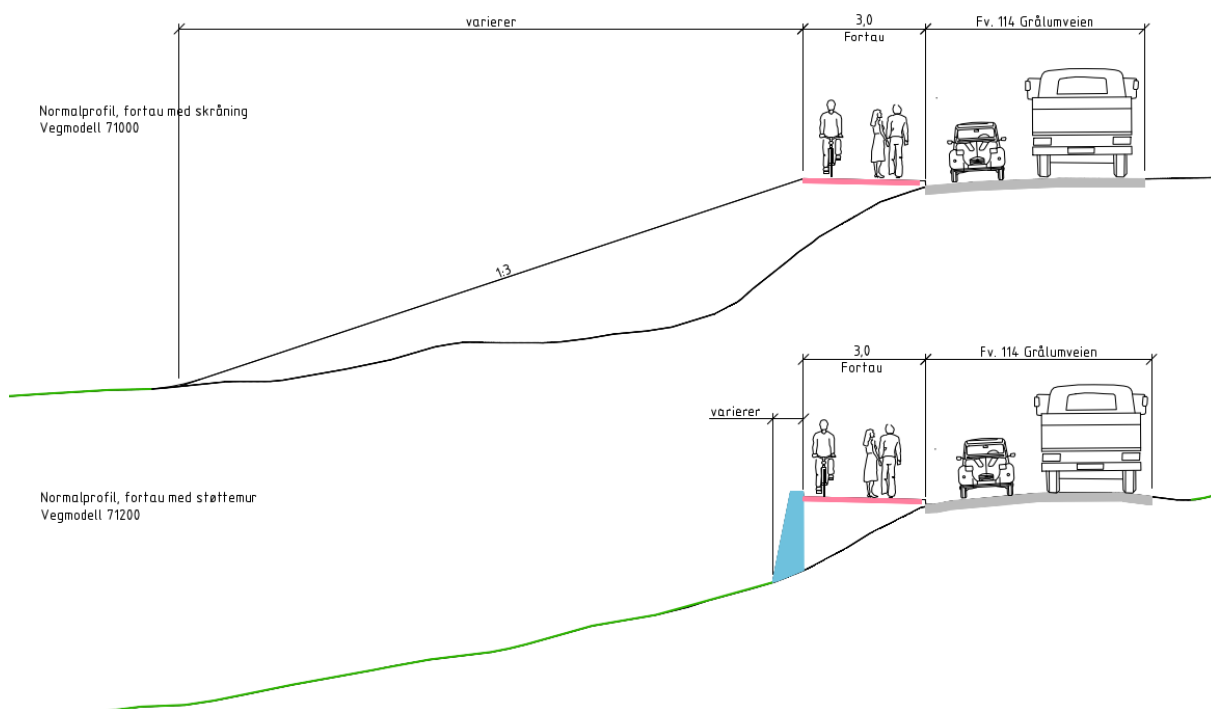
Figur 7-13: Normalprofil for alternativ 1 og 2. (Kilde: Østfold fylkeskommune)
