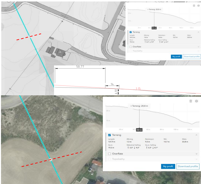
Figur 30: Terrangprofil fra Holandsveien og sørøst mot bunn av dalen. Rødstiplet linje indikerer grensen for 2*H unna skråningen ned til bunn av dalen.
