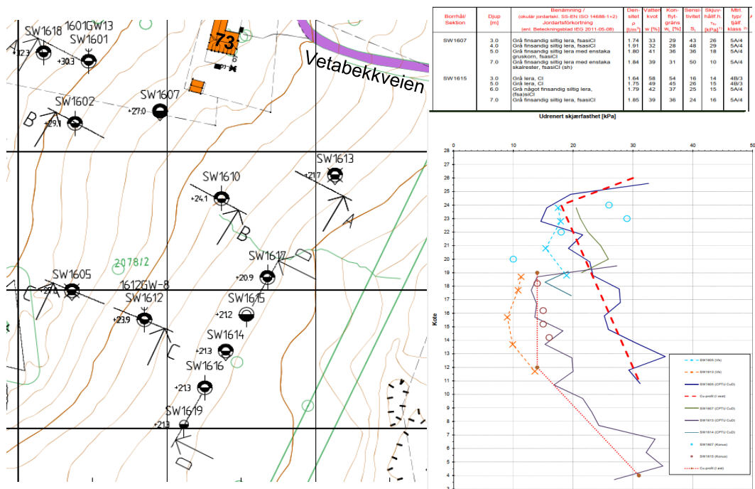
Figur 8: Borplan, resultater fra laboratorie og samlet CPTu-plot fra datarapport knyttet til Sweco-prosjekt som i dag går ved Holandsveien [3].
