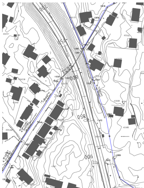
Figur 8-65: Eksisterende VA ved brulandkar på Kjøkkøy (Kilde: Sweco Norge AS)
