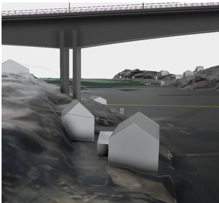
Figur 8-24 Utsnitt fra 3D-modell, viser søylene i akse 5. (Kilde: Sweco Norge AS)
